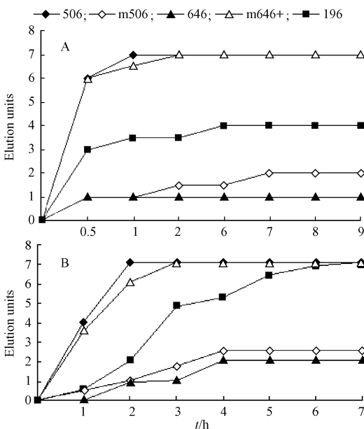
图 1 鸡(A)和豚鼠(B)红细胞解凝曲线
